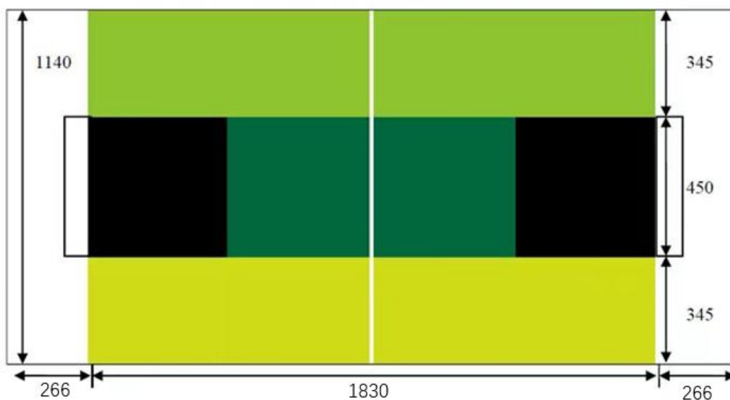
图 1.2 旧版比赛场地及尺寸 (mm)
