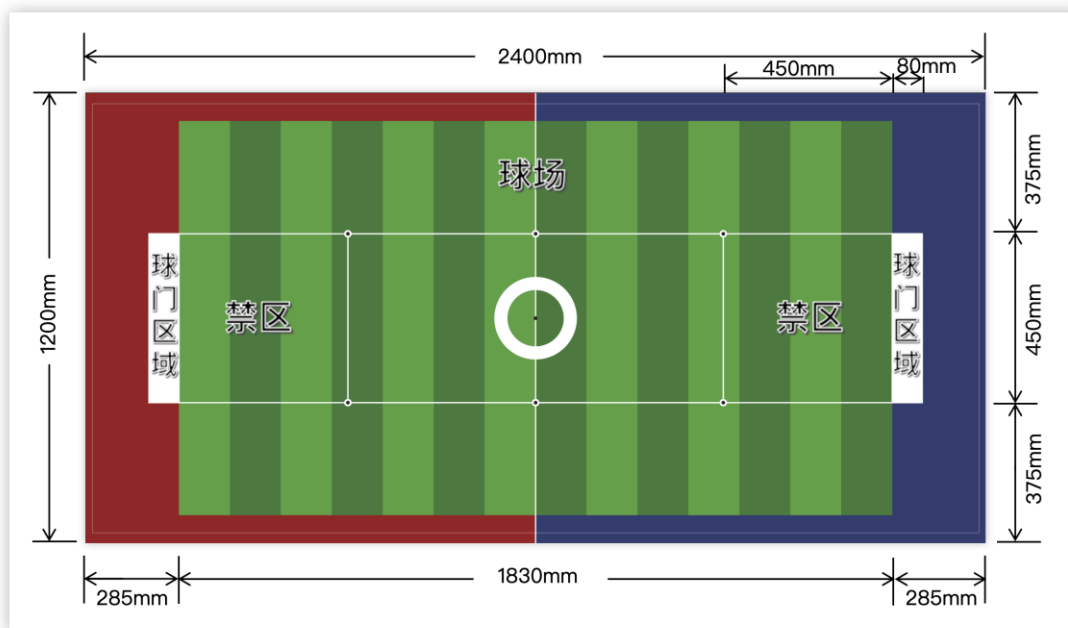
图 1.1 新版比赛场地及尺寸 (mm)
